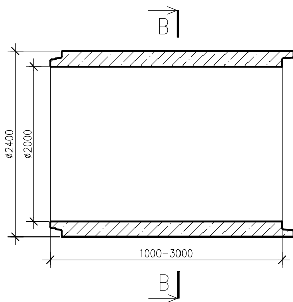
PRZEKRÓJ A-A
