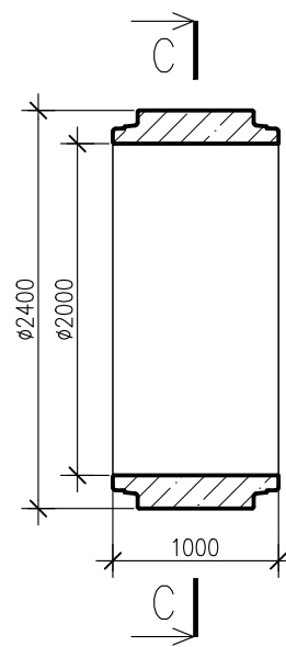
PRZEKRÓJ D-D
